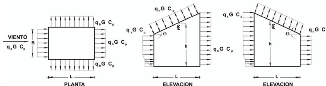
CUBIERTAS DE PENDIENTE UNICA (NOTA 4).
