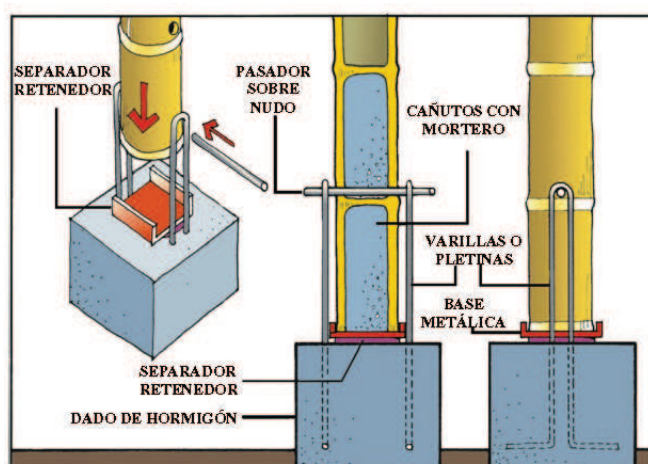
Figura E-B.1 Conexión cimiento – columna de guadua con separador en pletina
